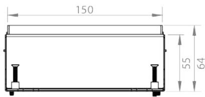
RVS S15ZR dekselset 15mm vloerinleg | zonder tapijtrand
