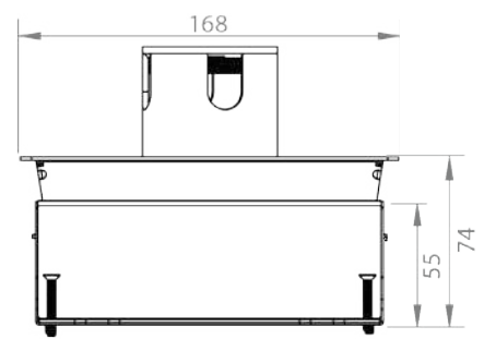
RVS S25 IP54 dekselset 25mm vloerinleg | tapijtrand
