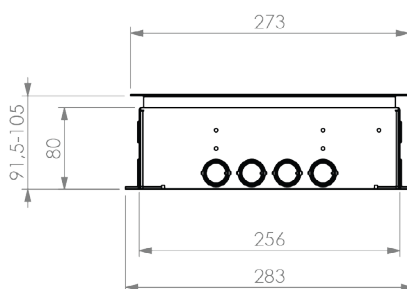
RVS T15 dekselset 15mm vloerinleg | tapijtrand
