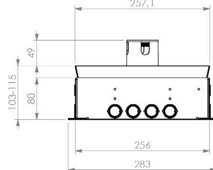
RVS T25ZR IP54 dekselset 25mm vloerinleg | zonder tapijtrand
