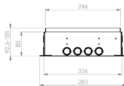
RVS T15ZR dekselset 15mm vloerinleg | zonder tapijtrand
