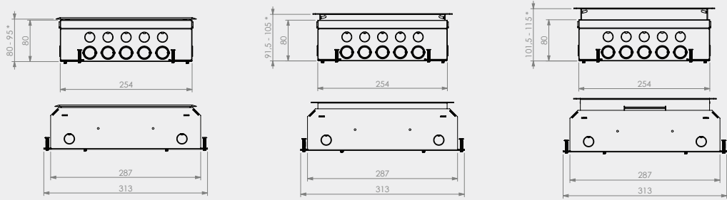
Dimensions avec couvercle rabattable T3 en synthétique Dimensions avec couvercle rabattable T15 en inox Dimensions avec couvercle rabattable T25 en inox
