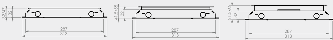
Dimensions avec couvercle rabattable T3 en synthétique Dimensions avec couvercle rabattable T15 en inox Dimensions avec couvercle rabattable T25 en inox
