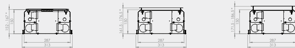
Dimensions avec couvercle rabattable T3 en synthétique Dimensions avec couvercle rabattable T15 en inox Dimensions avec couvercle rabattable T25 en inox
