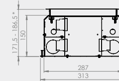
Maatvoering icm RVS T25 klapdeksel
