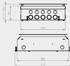
Maatvoering icm RVS T15 klapdeksel
