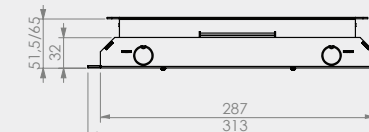
Maatvoering icm RVS T25 klapdeksel
