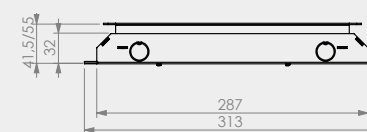
Maatvoering icm RVS T15 klapdeksel
