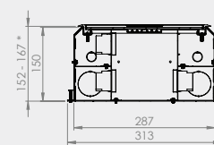
Maatvoering icm Kunststof T3 klapdeksel
