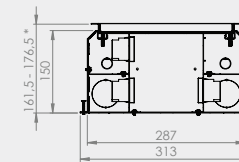
Maatvoering icm RVS T15 klapdeksel
