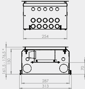
Maatvoering icm RVS T15 klapdeksel
