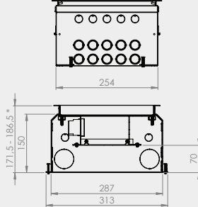
Maatvoering icm RVS T25 klapdeksel
