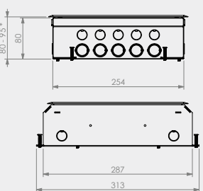
Maatvoering icm Kunststof T3 klapdeksel
