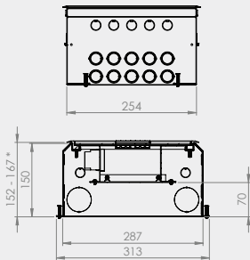
Maatvoering icm Kunststof T3 klapdeksel
