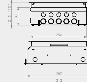
Maatvoering icm RVS T25 klapdeksel
