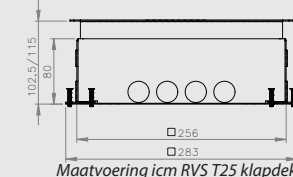
Maatvoering icm RVS T25 klapdeksel
