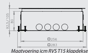
Maatvoering icm RVS T15 klapdeksel
