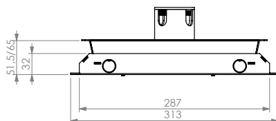
Jeu de couvercles T25 IP54 en inox Insert de sol 25 mm | Bord de tapis
