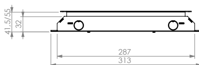
Jeu de couvercles T25ZR en inox Insert de sol 25 mm | Sans bord de tapis
