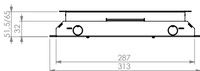
Jeu de couvercles T25 en inox Insert de sol 25 mm | Bord de tapis
