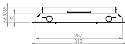
Jeu de couvercles T25ZR en inox Insert de sol 25 mm | Sans bord de tapis
