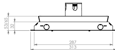
Jeu de couvercles T25ZR IP54 en inox Insert de sol 25 mm | Sans bord de tapis
