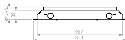
Jeu de couvercles T25ZR IP54 en inox Insert de sol 25 mm | Sans bord de tapis
