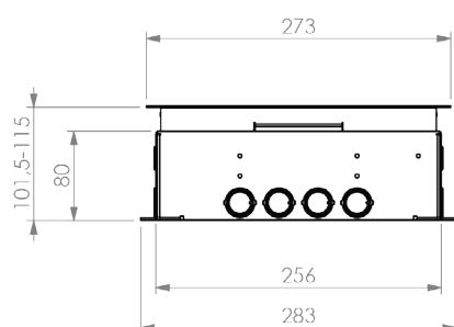
Jeu de couvercles T25 IP54 en inox Insert de sol 25 mm | Bord de tapis
