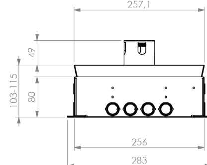
Jeu de couvercles T25ZR IP54 en inox Insert de sol 25 mm | Sans bord de tapis
