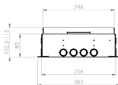
Jeu de couvercles T25ZR en inox Insert de sol 25 mm | Sans bord de tapis
